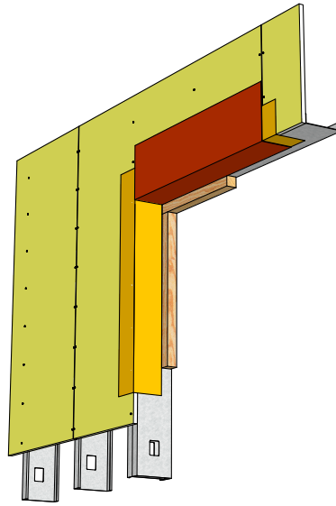
03. Metal trim
